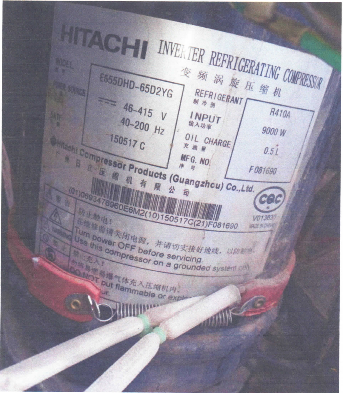
Değişimi yapılacak kompresör
